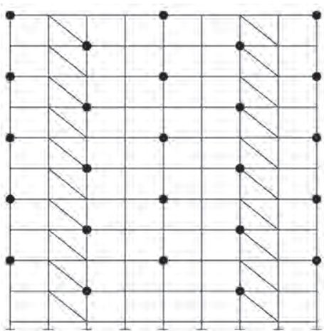
(D) Lines of Ties on Every Lift
